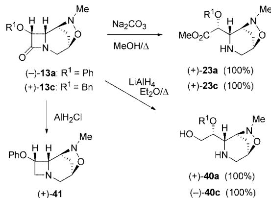
Scheme 14.
